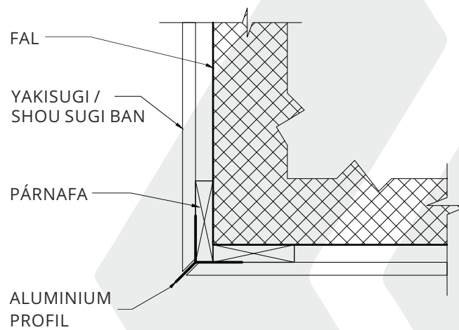
Ⓑ KÜLSŐ SAROK PROFILLAL
